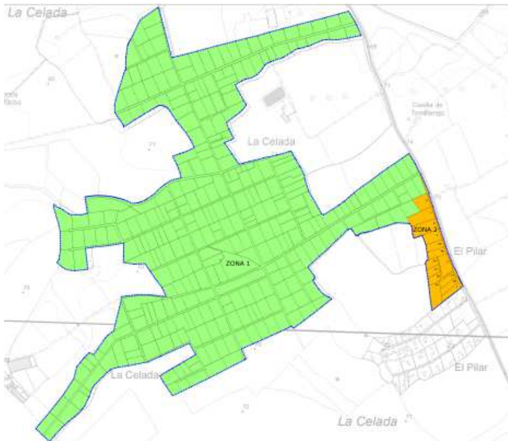
Delimitación de las dos Zonas de Ejecución que componen la Unidad de Ejecución (Plano O.1)
